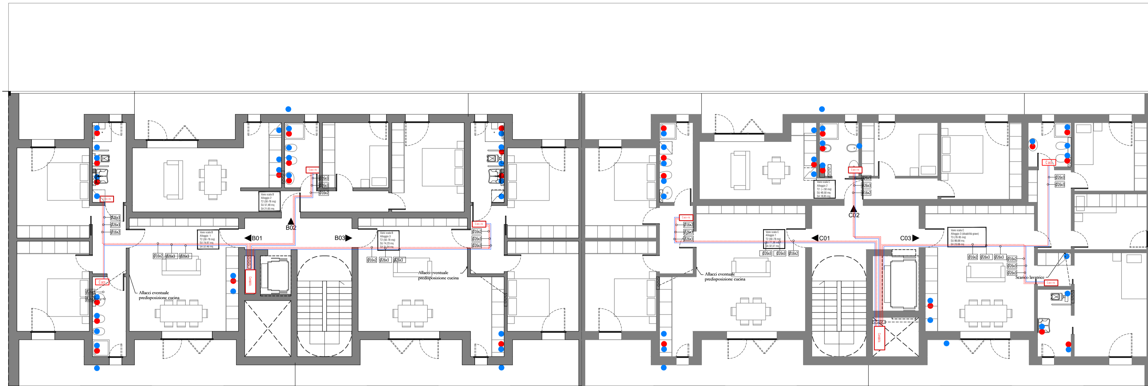
PIANTA PIANO PRIMO - SCALA B Scala 1:100
