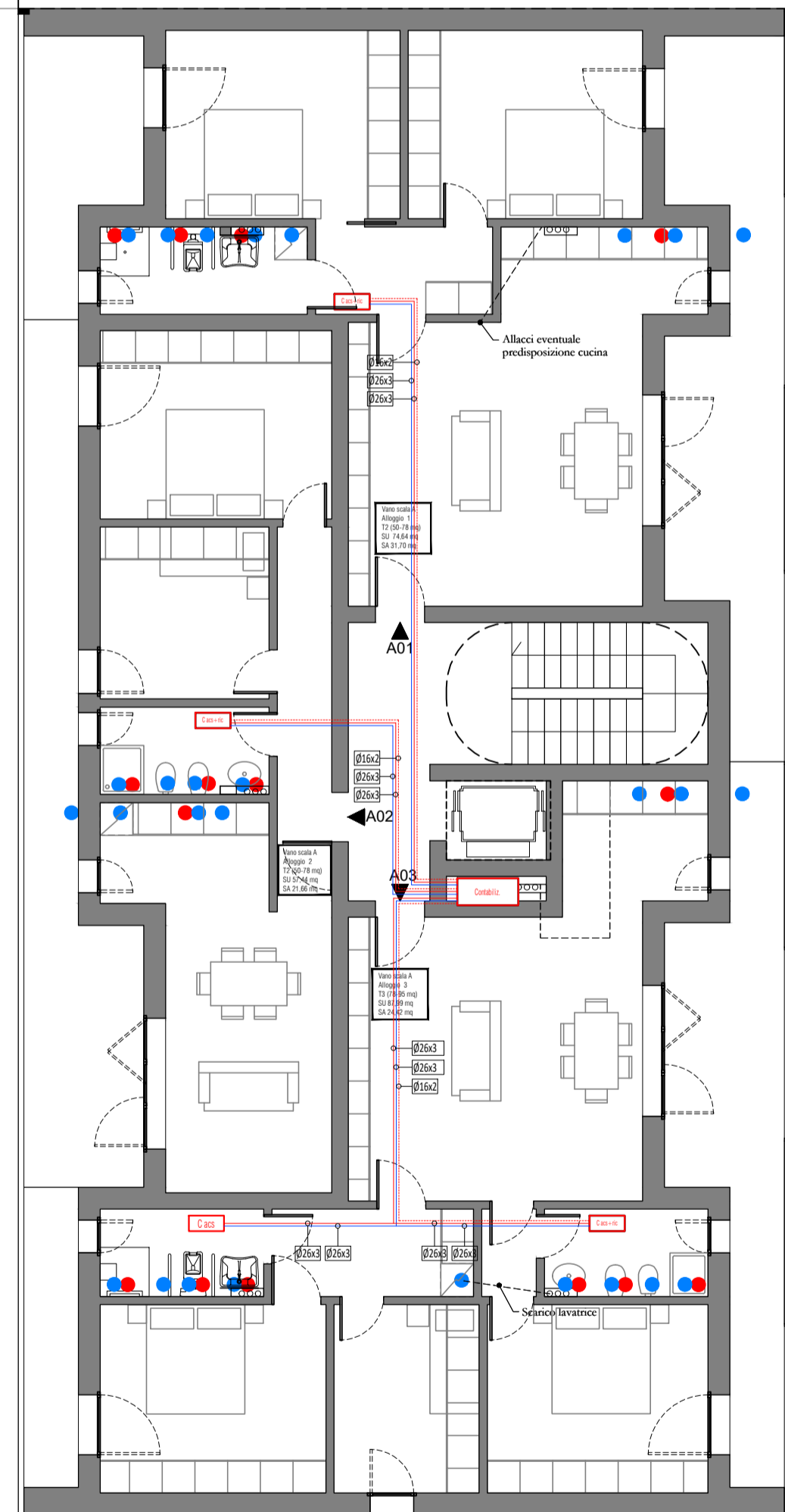
PIANTA PIANO PRIMO - SCALA A Scala 1:100
