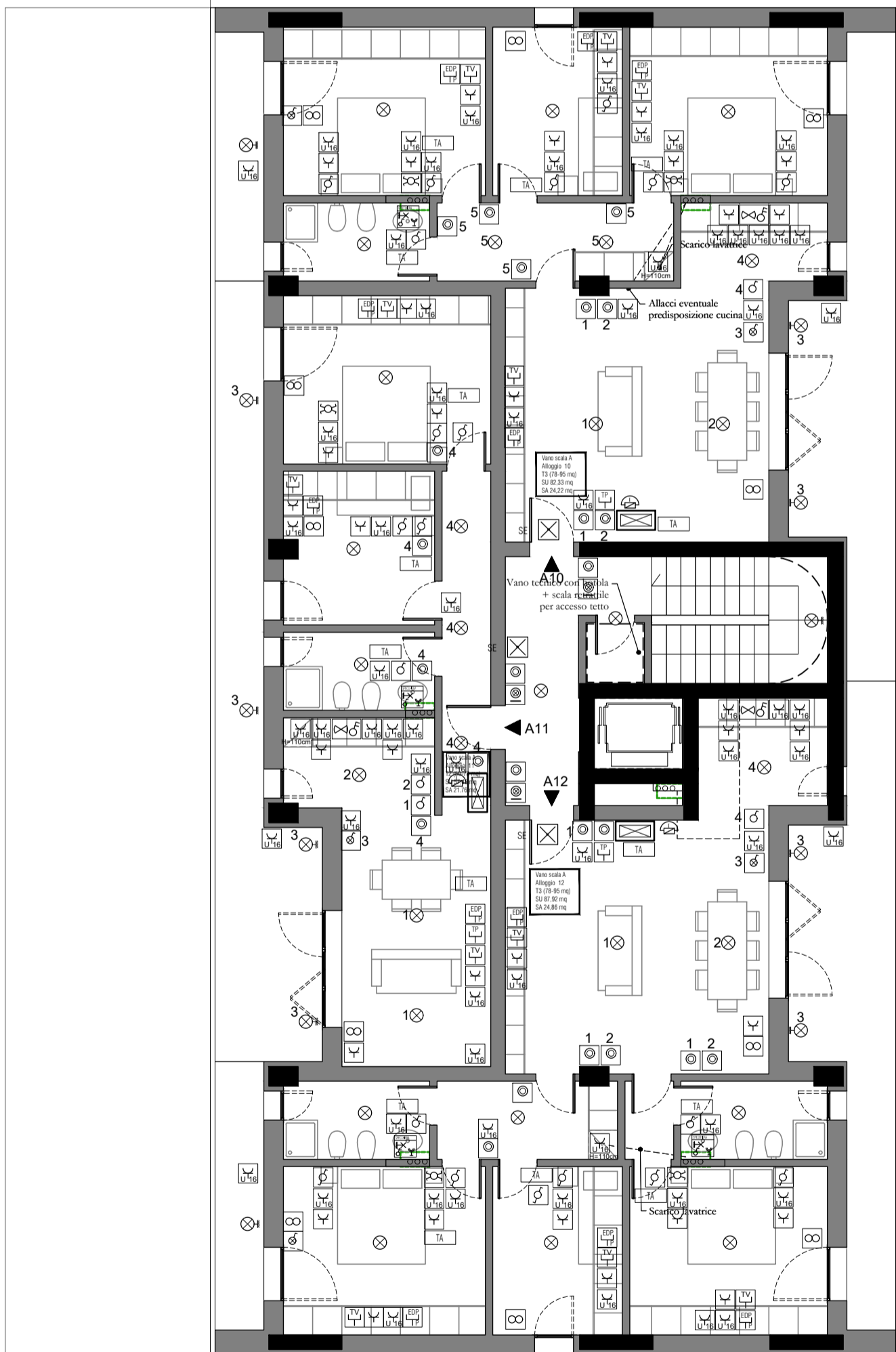
PIANTA PIANO QUARTO - SCALA A Scala 1:100
