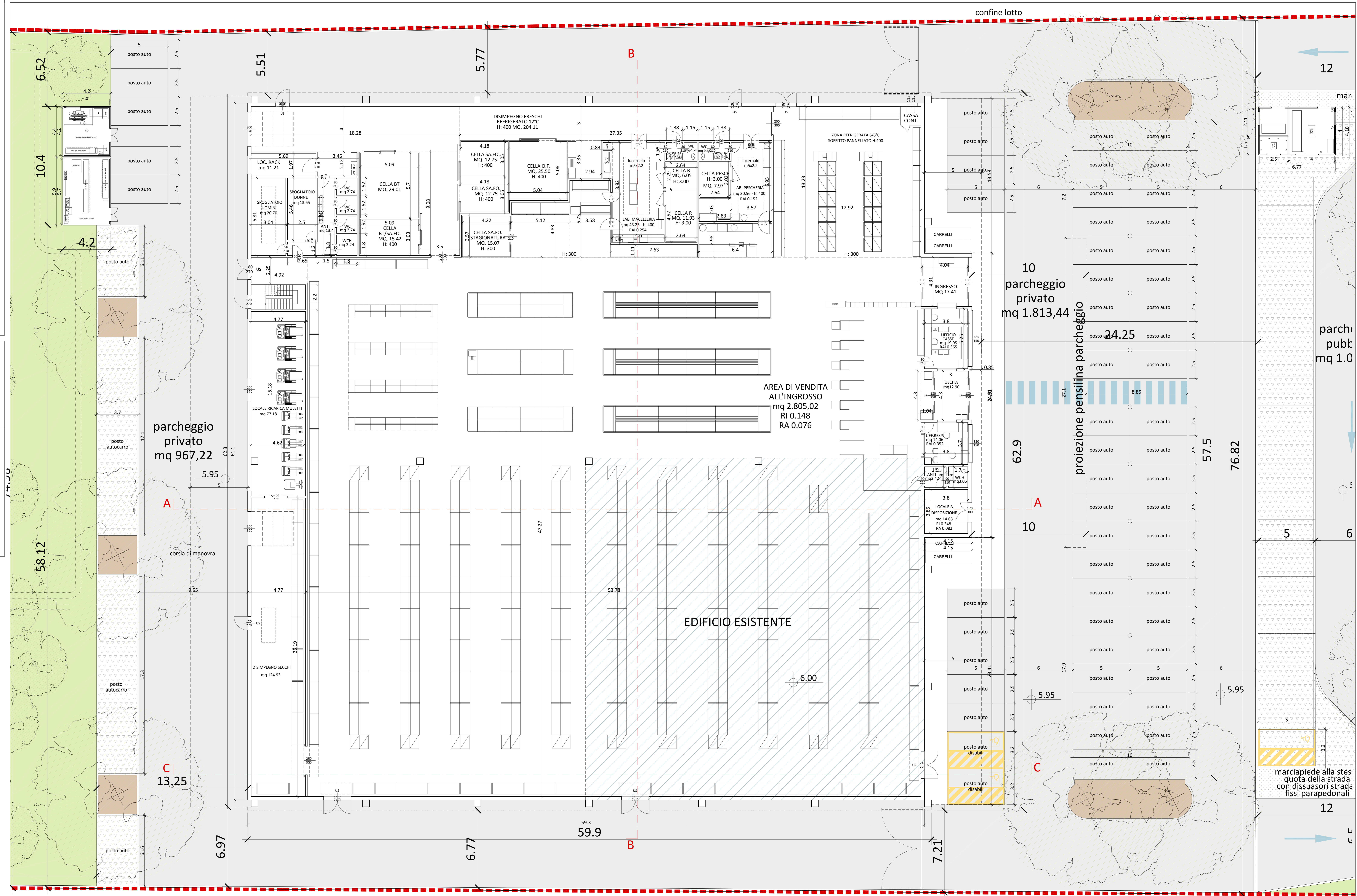
Pianta del piano terra
